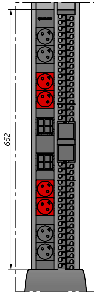
DETALLE A
